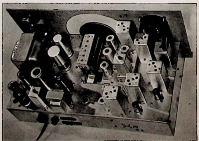
Abb. 4. Oben: Die übersichtliche Einzelteilanordnung auf dem Chassis Abb. 5. Links: Verdrahtungsansicht, Spulensatz von unten abgleichbar
