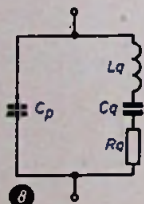
Abb. 8. Elektrisches Ersatzschaltbild eines Schwingquarzes
