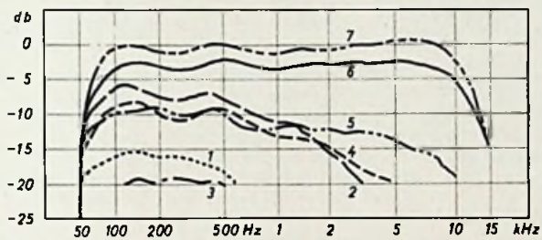
Abb. 3. Die Frequenzkurven der gleichen Bandsorten bei 19 cm/s
