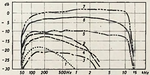
Abb. 4. Frequenzkurven bei geringerer Bandgeschwindigkeit von 9,5 cm/s
