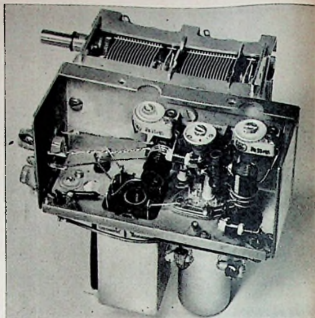
Links: Ansicht des bewährten UKW-Koffers „Noraphon-Ultra“ von Nora. Daneben: Ansicht und (ganz rechts) Blick in den UKW-Teil des Schaub-Reisesupers „Camping“
