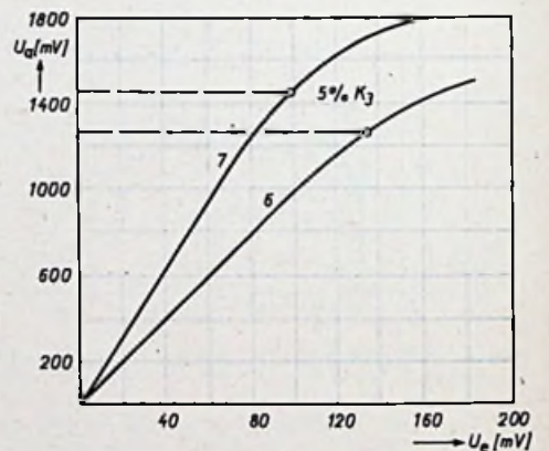
Abb. 6. Ausgangsspannung in Abhängigkeit von der Aussteuerung bei 19 cm/s Bandgeschwindigkeit für das Band 6 (LGH) und das Band 7 (LGS)
