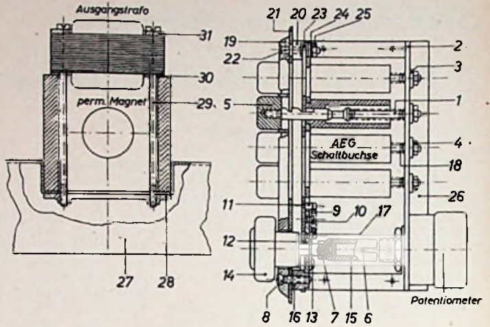
Eine schematische Zeichnung zur Montage des Ausgangsrafos
