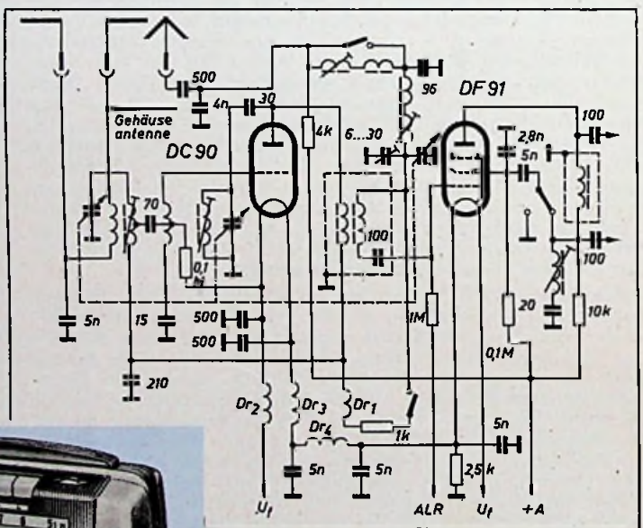
Koffersuper „Pinguin“ mit den Bereichen UKW, MW, LW (Akkord-Radio)
