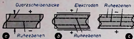
Abb. 7. Schwingungsformen von Oberwellenquarzen (Dickenschwinger). a = Grundschwingung in einer Halbphase; b = zweite Harmonische, nicht anregbar, da Elektroden gleiche Polarität aufweisen; c = dritte Harmonische, ist anregbar
