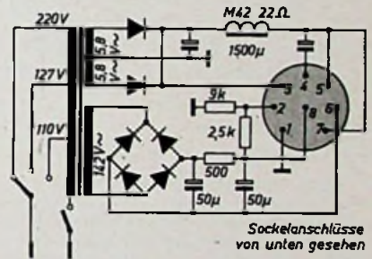
Schaltung des „Babyphon“ von Metz. Der Batterieersatz (links) und Netzzusatz (rechts)
