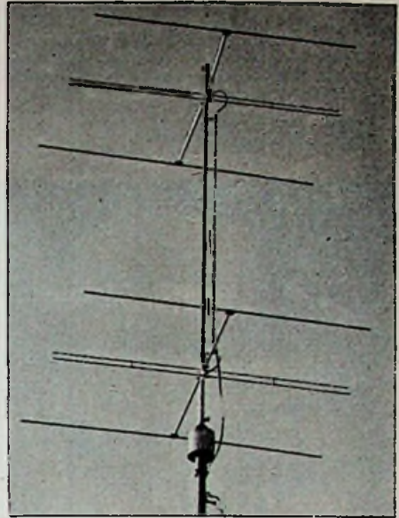
Zweiebenen-UKW-Antenne „2 x D 510“, auf Antennenrotor aufgebaut (Kathrein)
