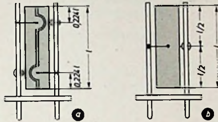
Abb. 3. Montage von Quarzschwingern im Halter; a = Biegeschwinger, b = Längsschwinger
