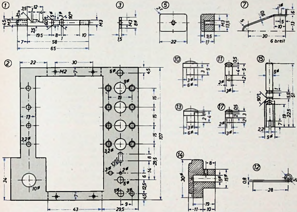
Bauzeichnungen für den Rahmen des Drucktastenaggregates 2 und die Zubehörteile
