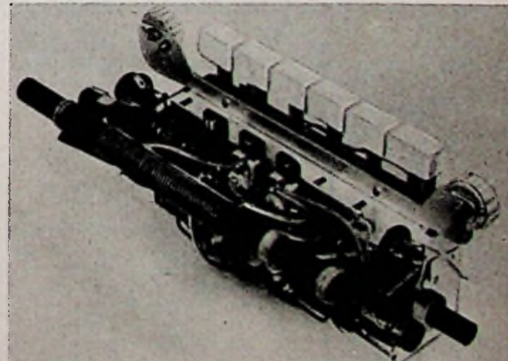
Kombination von Tastenschalter sowie AM-Eingang- und Oszillatorteil im Lorenz-„Touring“
