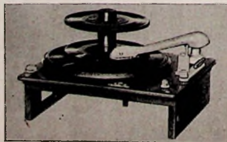
Dreitouren-10-Platten-Spieler „Rex A“ mit Spezial-Abwurfachse (Perpetuum-Ebner)
