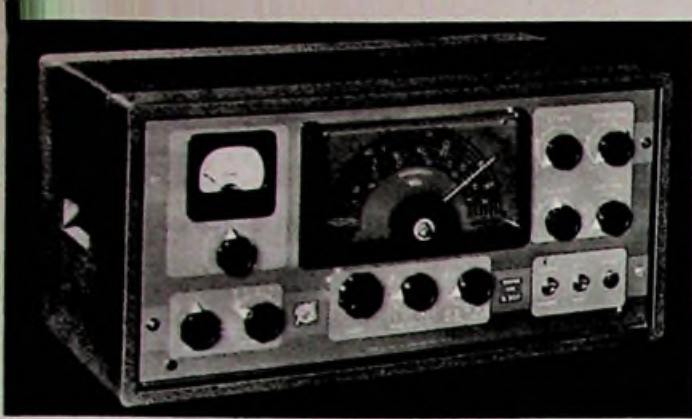
Abb. 3. Vorderansicht des Amateur-Doppelsupers. Auf der Frontplatte sind die zusammengehörigen Bedienungsriffe auch optisch zusammengefaßt
