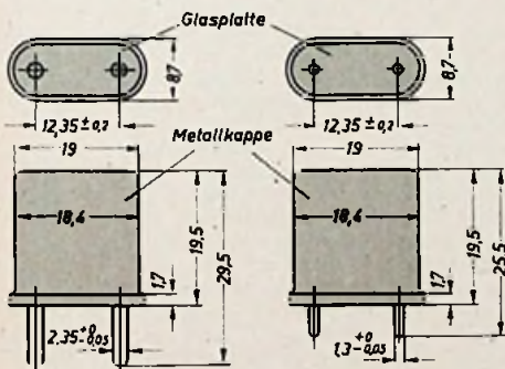
Abb. 1. Abmessungen des Standard-Quarzhalters
