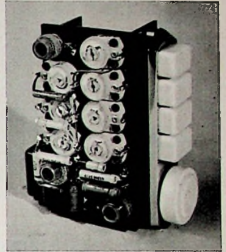
Abgleichseite des fertigen Drucktastenaggregates mit den Trimmern und Spulen
