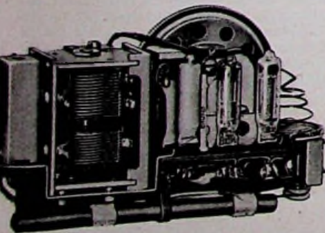
V. l. n. r.: Der raffinierte Innenaufbau des kleinen Grundig-Taschensupers „Mini-Boy“ (rechts im Foto sind drei von den vier Subminiaturröhren erkennbar, links davon der Doppeldrehko, daneben ein ZF-Bandfilter und ganz rechts eine Feder zum Festhalten der Heizbatterie; rechts hinten sitzt der Lautsprecher und unten die Ferritstabantenne). Ansicht und Stromversorgung des Grundig-„UKW-Boy“
