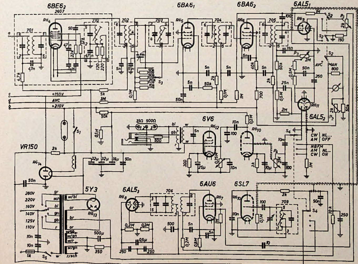
Abb. 2. Unten: Gesamtschaltung des Doppelsupers
