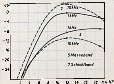
Abb. 1. Die Empfindlichkeit (Ausgangsspannung) bei 1 kHz und 10 kHz in Abhängigkeit von der HF-Vormagnetisierung
