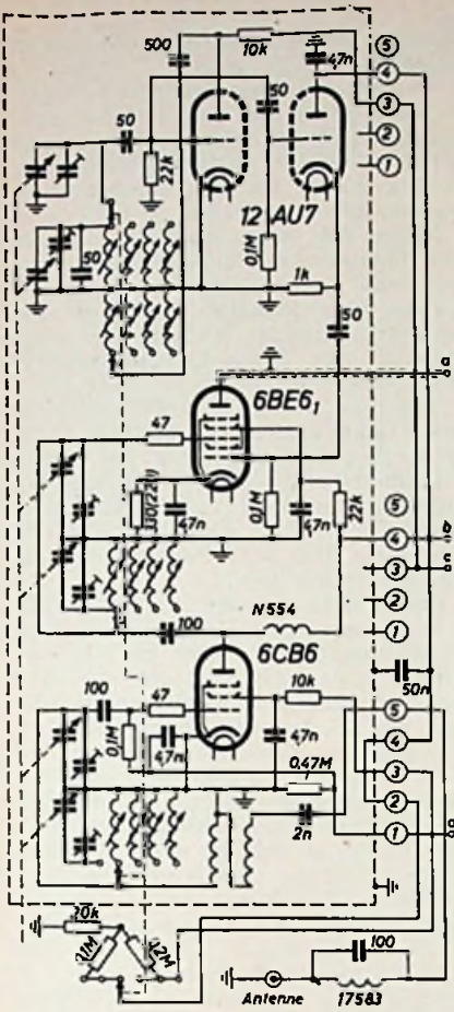
Abb. 1. Schaltung des HF-Eingangsteiles. Punkte a ... d sind Verbindungen zum ZF- und Netzteil
