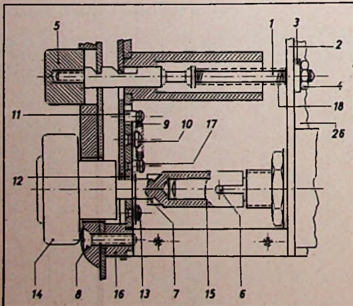
Die Verdrahtung ist rüttelsicher an einer Lötösenplatte festgelegt. Links neben dem Potentiometer sieht man die Koaxbuchse und Listkupplung
