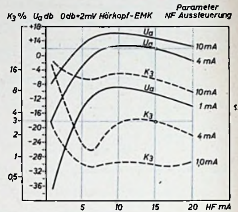
Abb. 5. Ausgangsspannung und Klirrfaktor in Abhängigkeit von der HF-Vormagnetisierung eines LGN-Bandes
