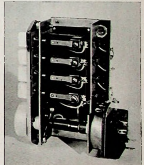
Über dem Lautstärkereglers (unten) erkennt man die aus Schaltbuchsen hergestellten Drucktasten
