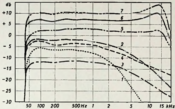
Abb. 2. Verschiedene Frequenzkurven bei hoher Bandgeschwindigkeit 76,2 cm/s
