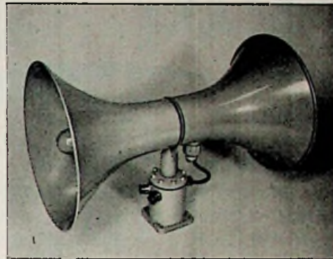
Ultratron-Hochleistungs-Doppeltrichter-Lautsprecher mit Druckkammersystem (12 W), montiert auf einem wasserdicht gekapselten Transformator
