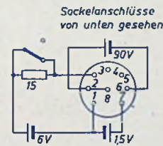
Schaltung des „Babyphon“ von Metz. Der Batterieersatz (links) und Netzzusatz (rechts)
