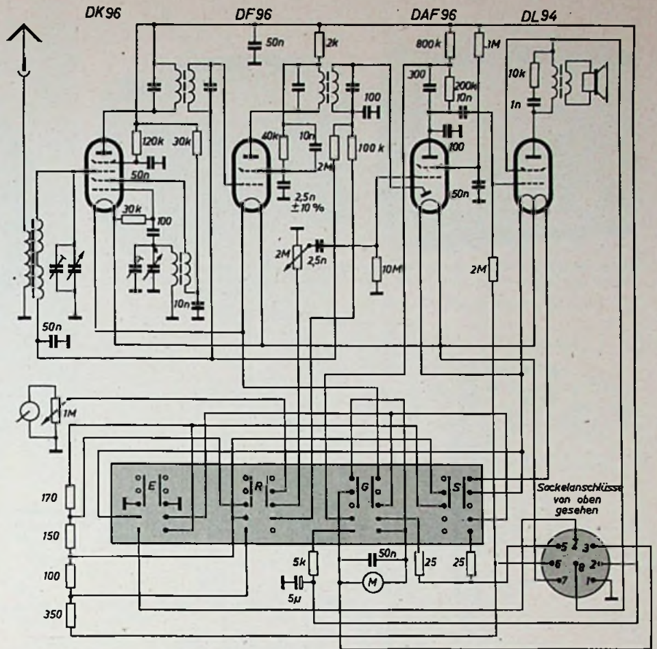
Schaltung des „Babyphon“ von Metz. Der Batterieersatz (links) und Netzzusatz (rechts)
