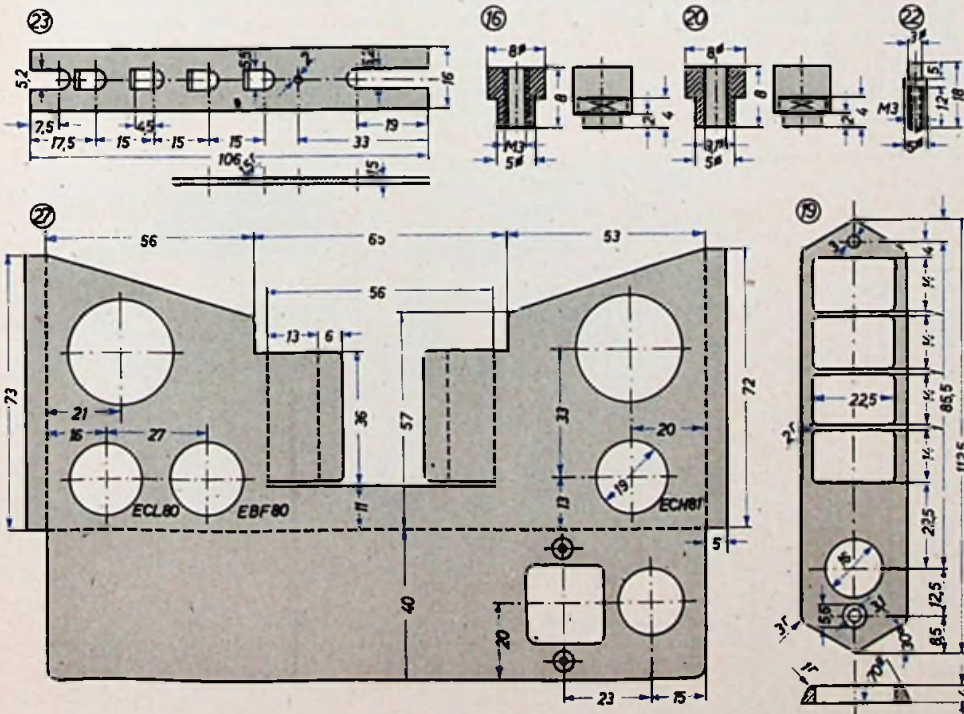
Aufluß für das Chassisblech 27, die Drucktastenabdeckung 19 usw.; Pos. 23 ist das Sperrblech
