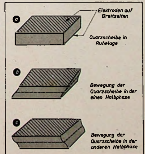
Abb. 6 (unten). Scherbewegungen von Dickenschwinger-Quarzen
