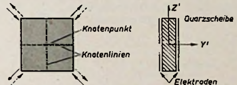
Abb. 4. Bewegungsformen des Flächenschwingers
